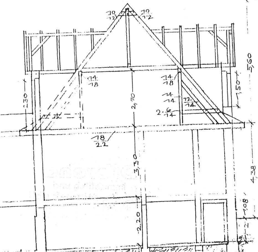
Seitenansicht
