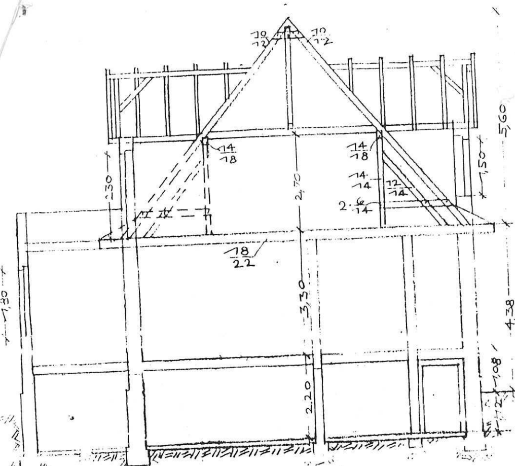
Schnitt a-b
