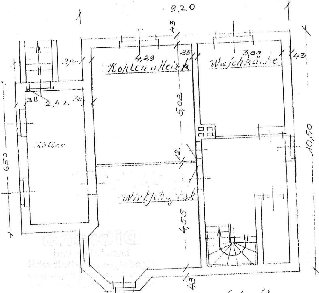
Kellergeschoß
