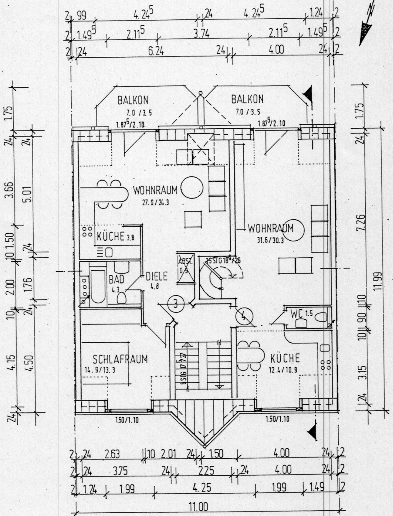
DACHGESCHOSS M1:100
