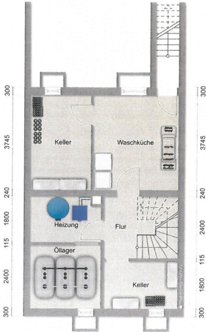
Keller
