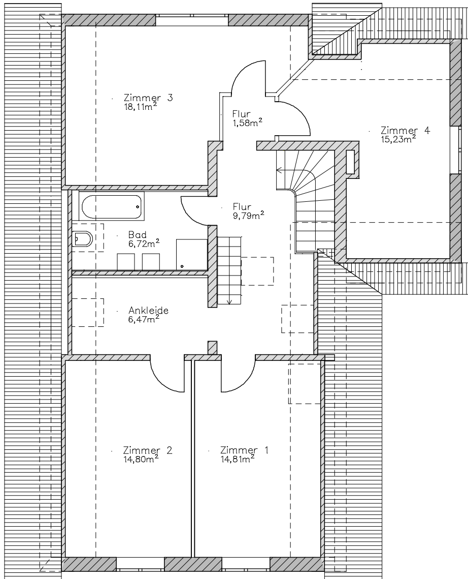
Grundriss DG
