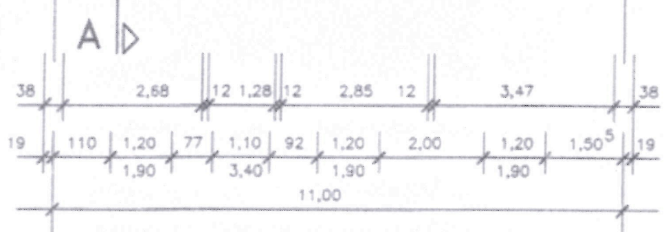
ERDGESCHOSS
