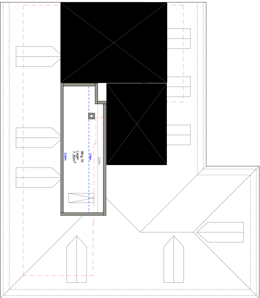
Dachboden BESTAND
