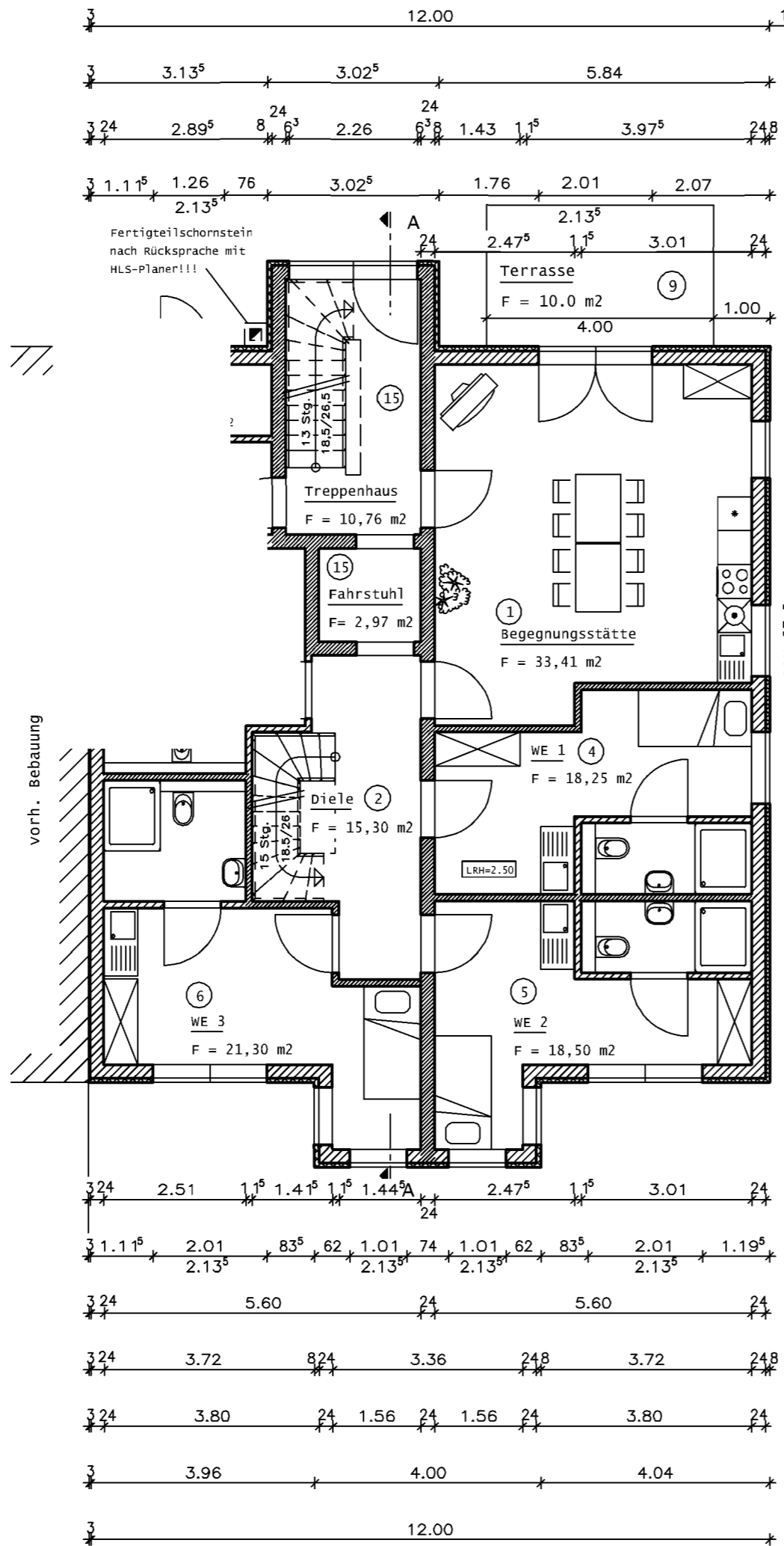
Grundriss EG
