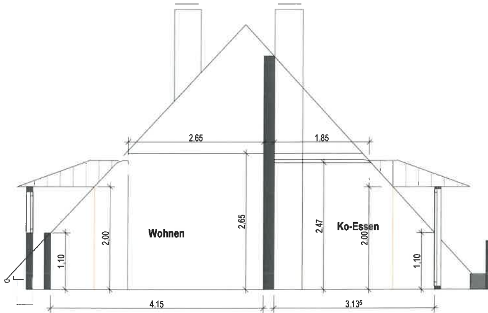
Schema-Schnitt
