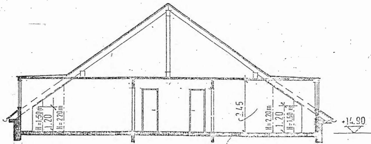
B-B
