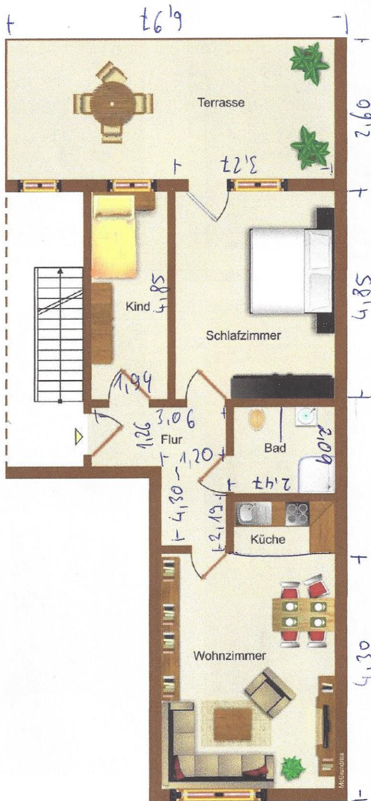
Grundriss 3,78
