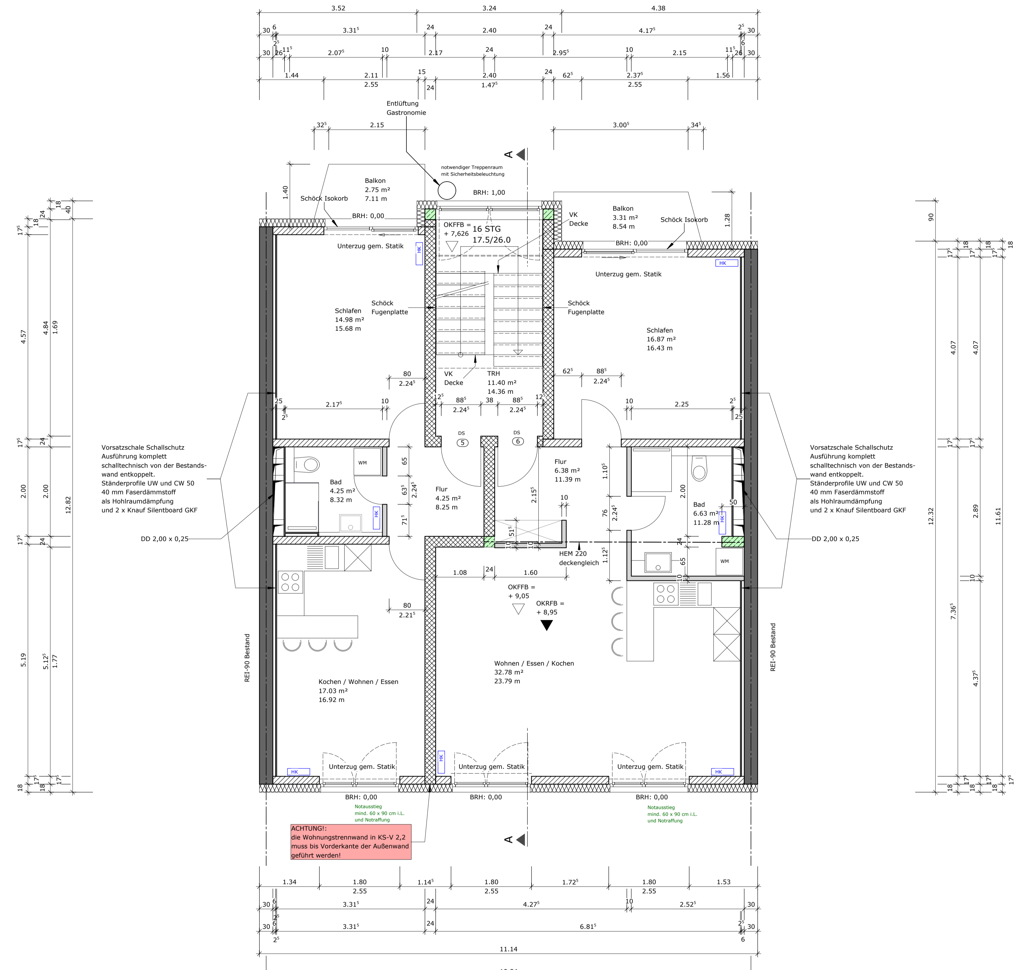
GRUNDRISS 3.OG 1:50
