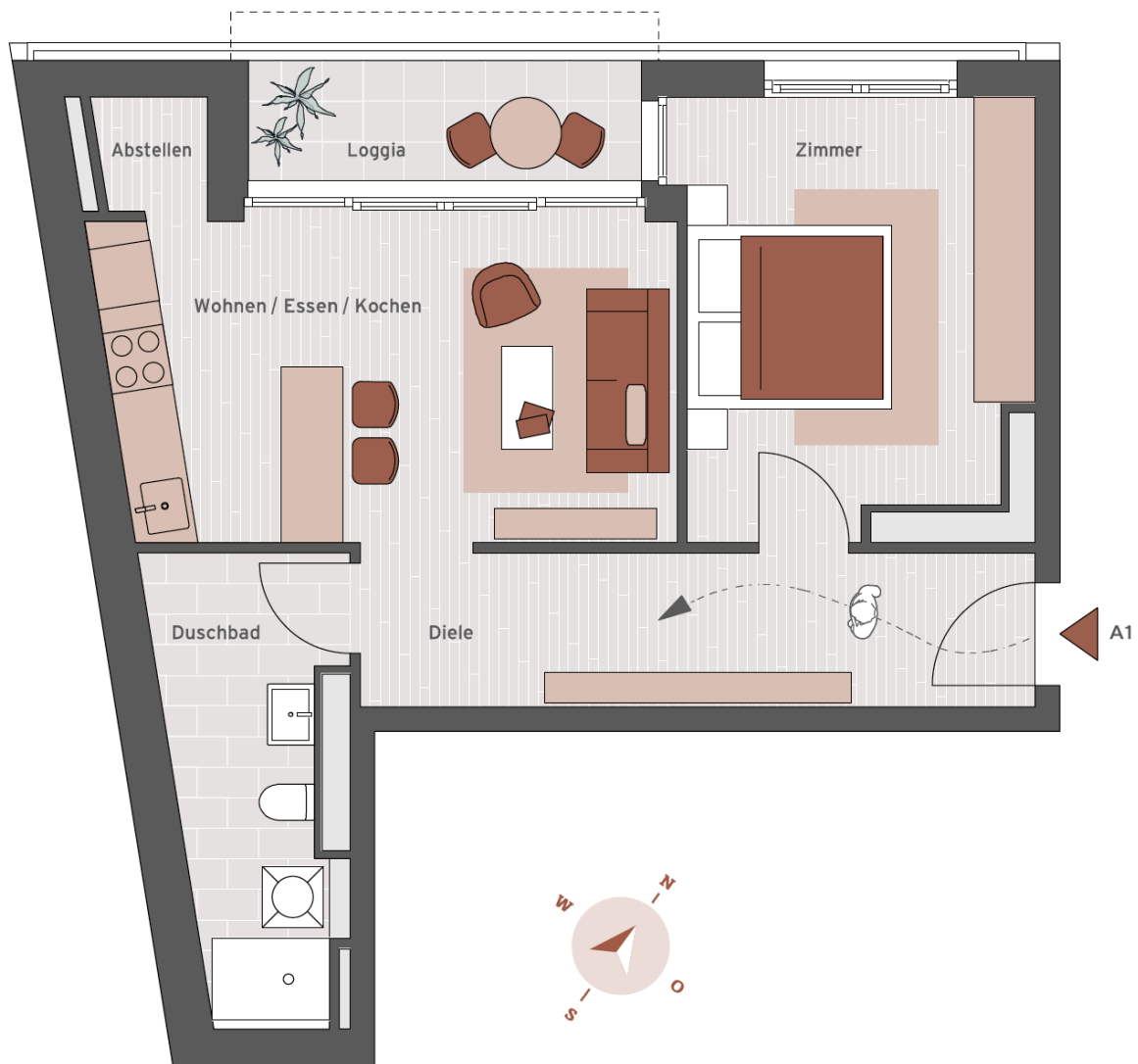
Grundriss 2-Zimmer-Wohnung Niddagastrasse 32, 53 qm
