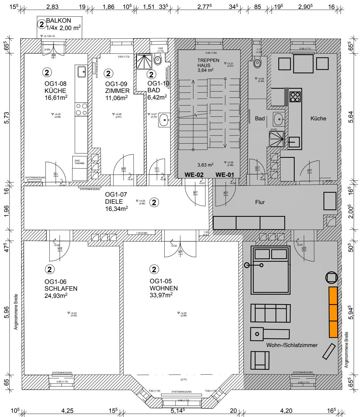
1. Obergeschoß 1:100
